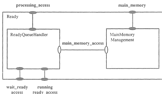
Figura 8 Arquitetura LOTOS de Ready
