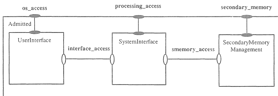
Figura 6 Arquitetura LOTOS de Admitted
